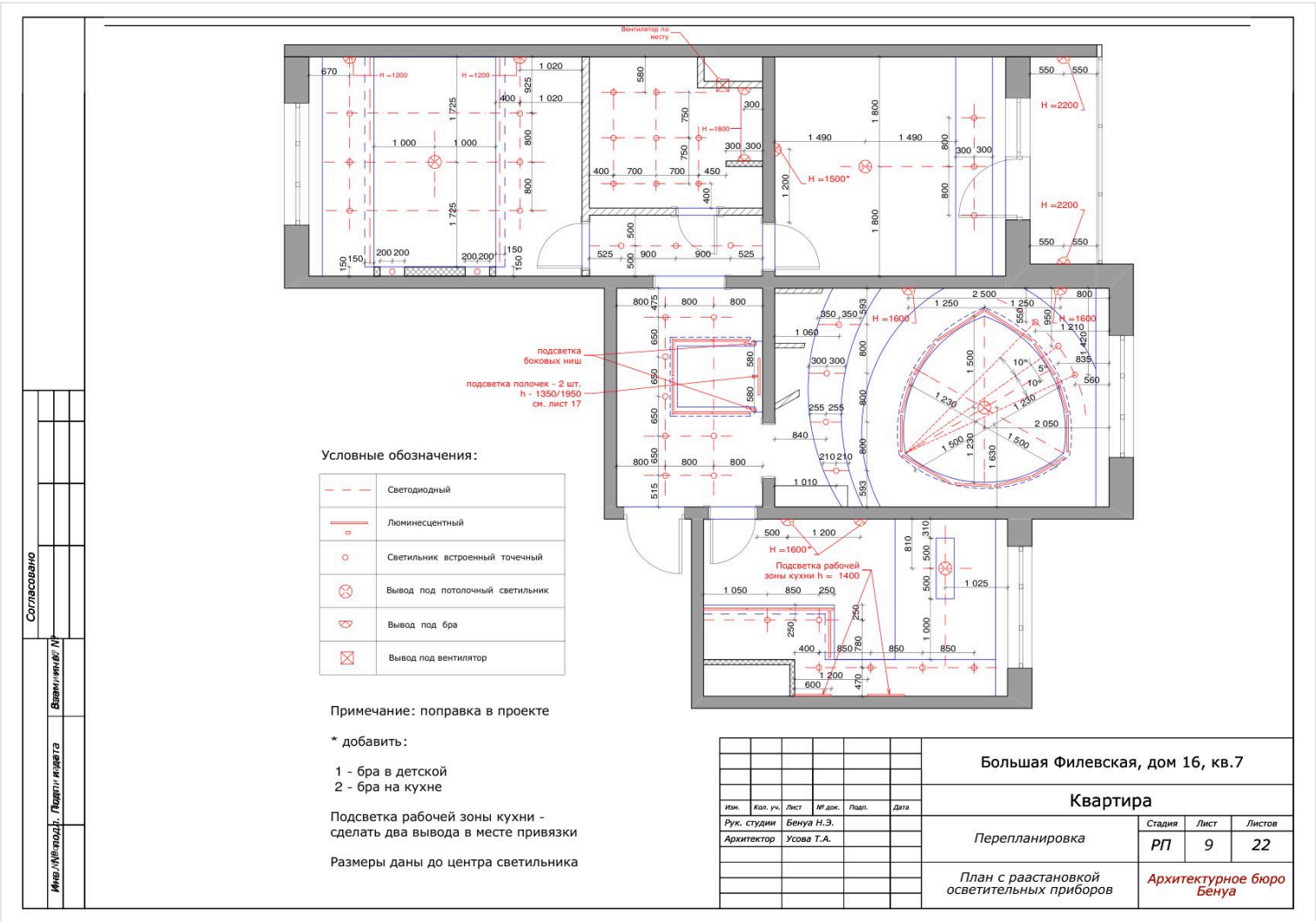
План расстановки осветительных приборов
