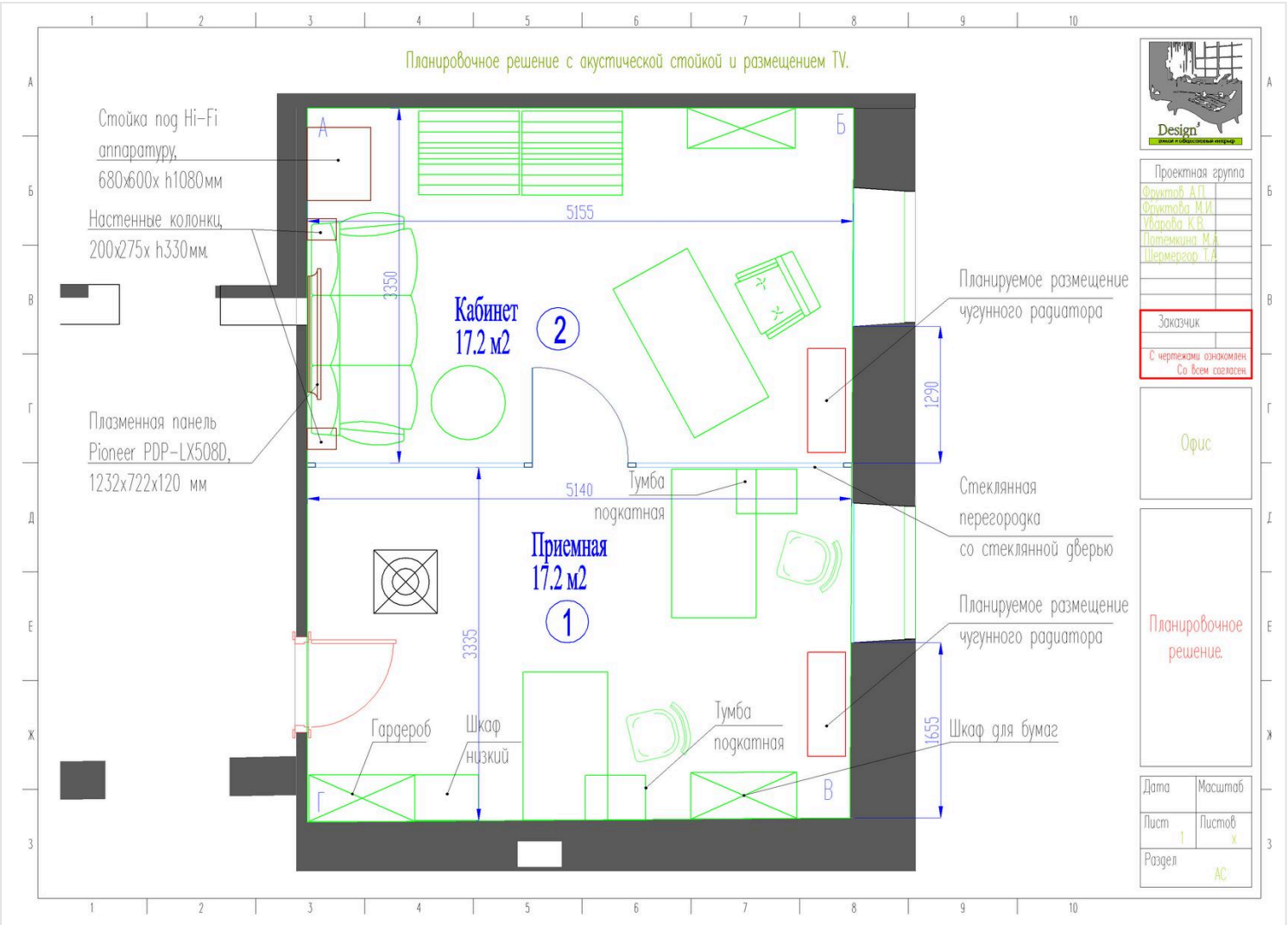
Планировочное решение кабинета и приёмной
