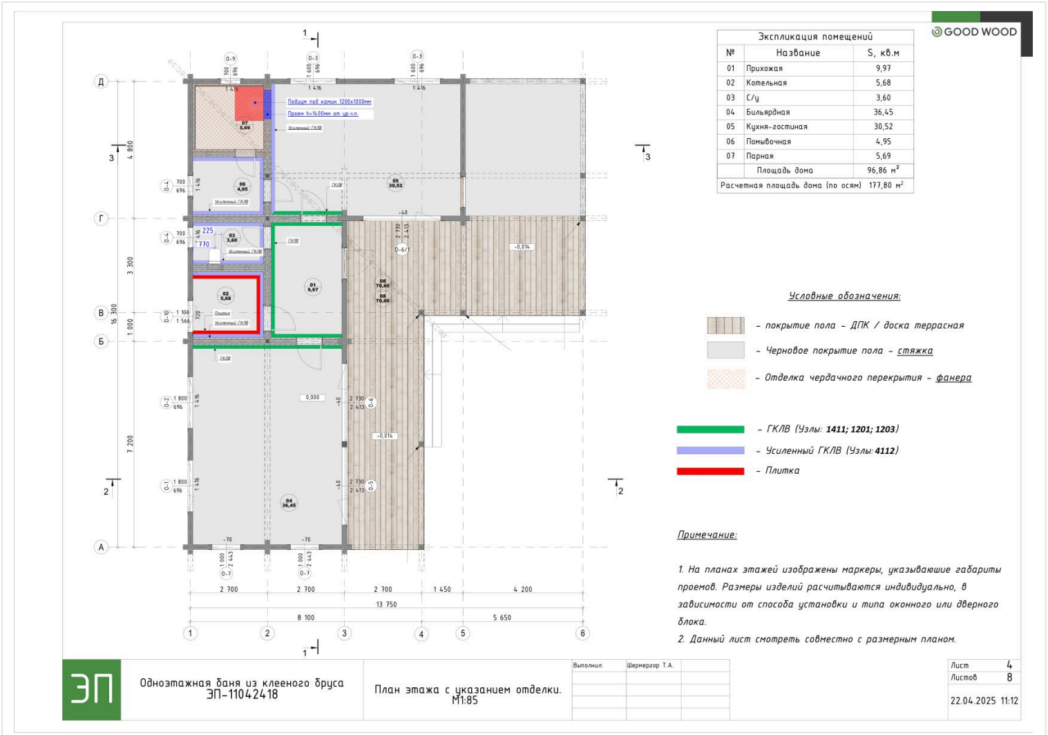
План этажа с отделкой
