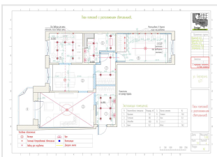
План потолков с размещением светильников
