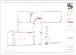
План демонтажа перегородок
