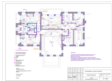
План осветительной сети 2 этажа
