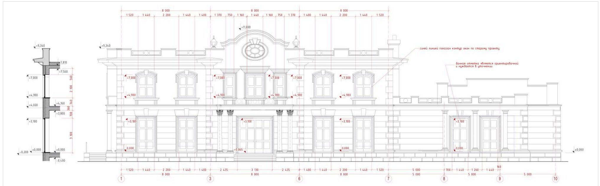
Фасад главный
