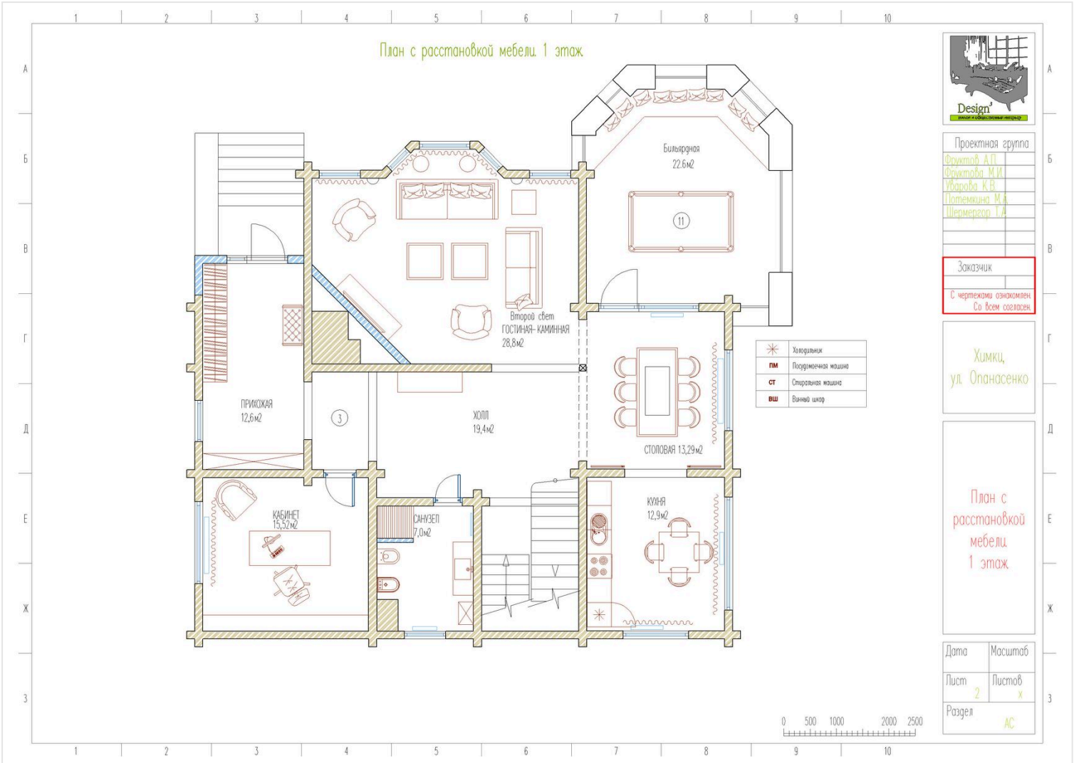
План расстановки мебели, 1 этаж
