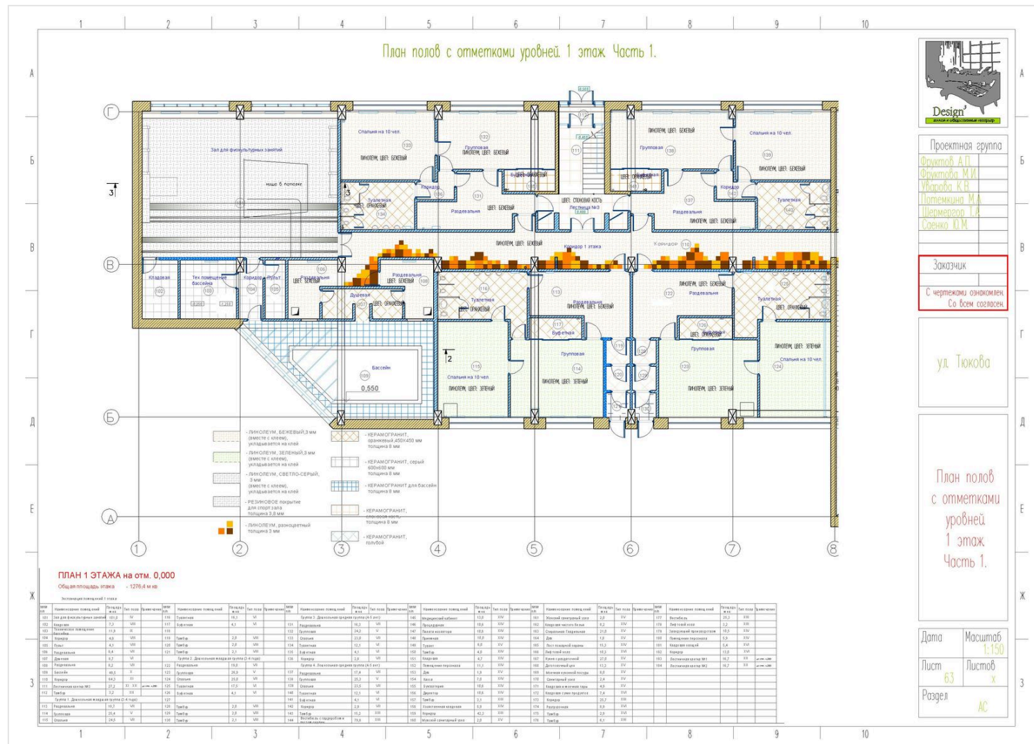
План полов с отметками уровней, 1 этаж, часть 1
