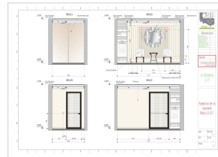
Развёртки стен, прихожая
