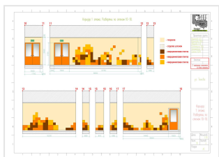
Развёртки стен коридора 1 этажа, 10-18
