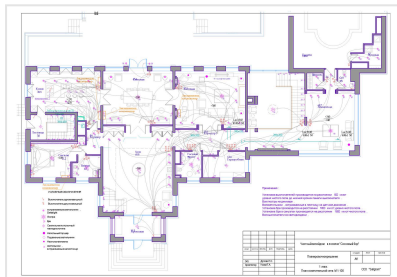
План осветительной сети 1 этажа
