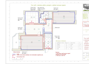
План полов с раскладкой покрытий
