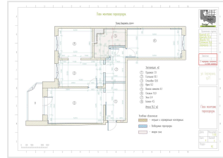
План монтажа перегородок
